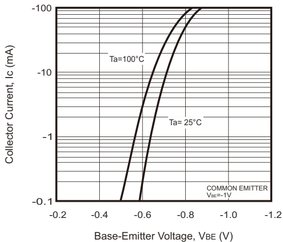
Fig.5 - I_c - V_{BE}
