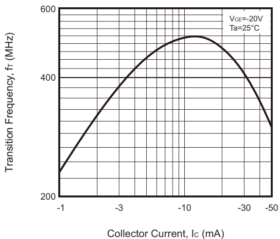
Fig.7 - F_T - I_c
